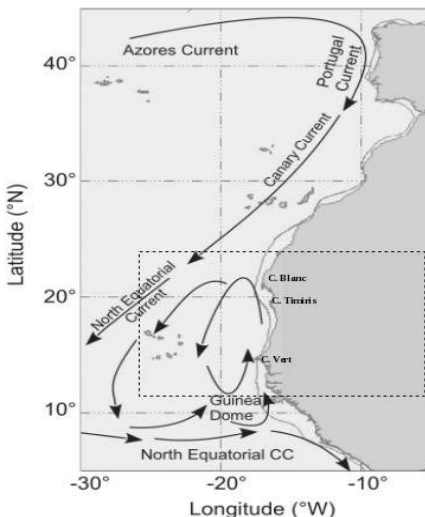
Figure 1.5 – Carte schématique de la zone d'étude (cadre en tireté), incluant la péninsule Ibérique et la région d'upwelling Nord-Ouest Africain et ces principaux courants de surface : les courants des Açores et du Portugal, le Courant Nord Equatorial et le Contre Courant Nord Equatorial. L'isobathe 200 m est indiquée en ligne continue. (adaptée de, Benazzouz et al., 2014).
