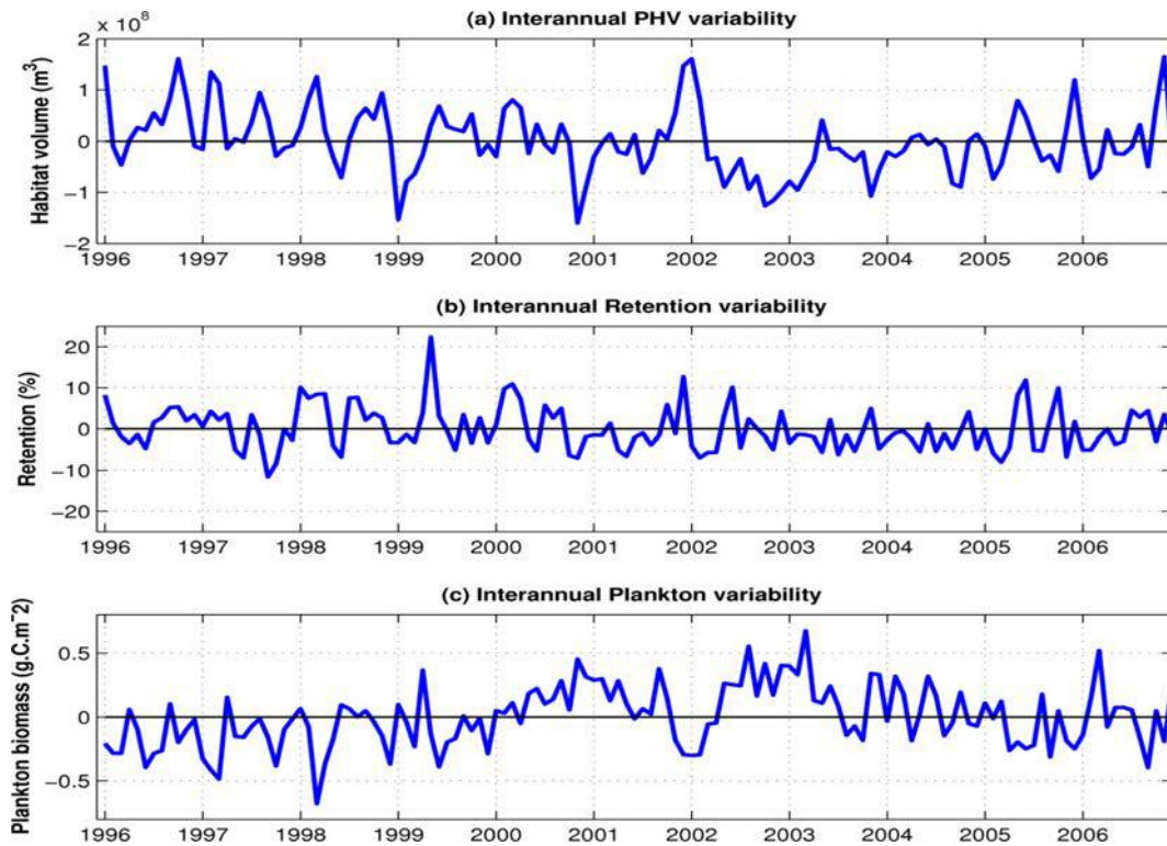
Figure 4.14 – Anomalies du (a) volume d'habitat de ponte ( m^3 ), (b) de la rétention (%) et (c) de la biomasse totale de plancton ( g.C.m^{-2} ) moyennées dans la zone sénégalo-mauritanienne. La ligne noire correspond à la délimitation de la valeur zéro.
