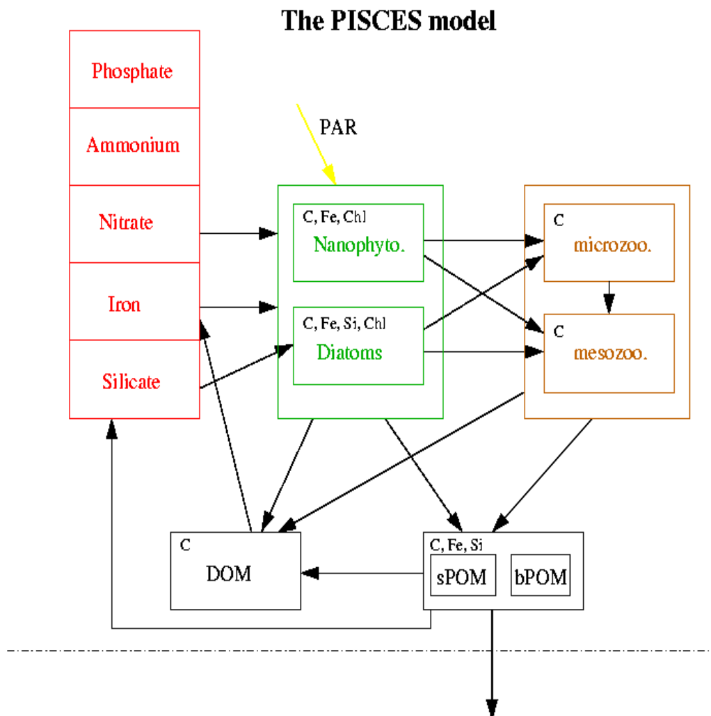
Figure 2.4 – Description schématique de la structure du modèle d'écosystème PISCES (Aumont and Bopp, 2006). En rouge les nutriments; en vert, le phytoplancton, en orange, le zooplancton; en noir, les détritrus.
