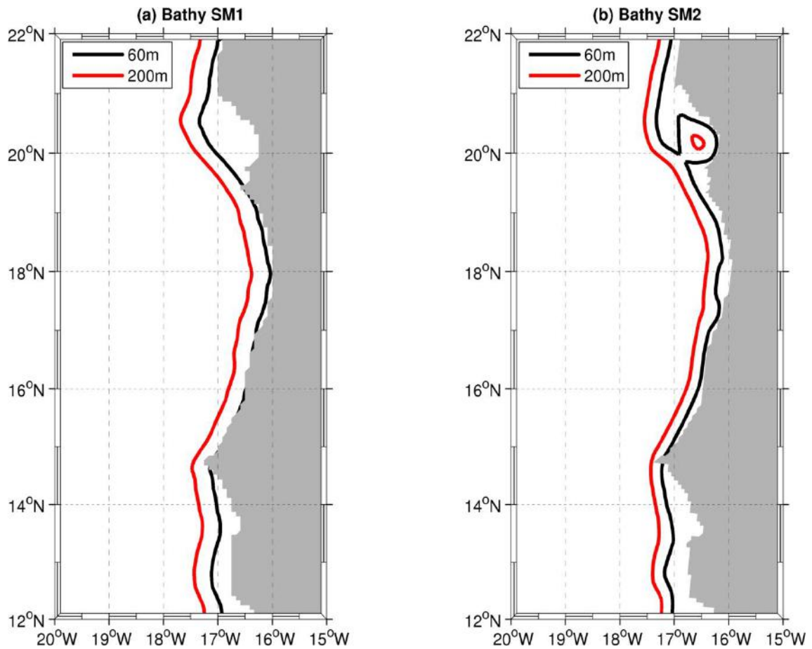
Figure A.1 – Profil spatiale de Bathymetrie pour les configurations ROMS (a) SM1 and (b) SM2 (right). Les isobathes 60m (ligne en noire) et 200 m (rouge) sont superposées. La cavité dans SM2.
